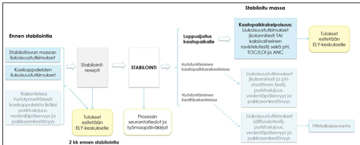
Kuva 3. Stabiilointi- ja kiinteytysprosessi ja sen laadunvarmistus.
